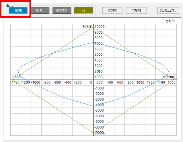
柱脚長期許容耐力曲線
