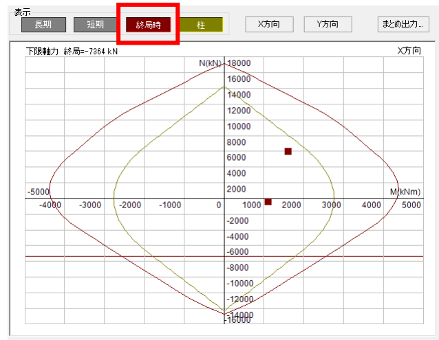
柱脚終局耐力曲線
