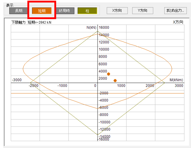
柱脚短期許容耐力曲線
